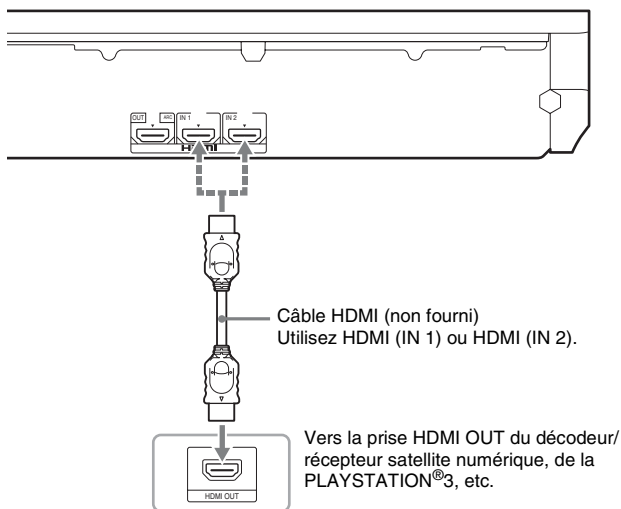
Panneau arrière de l'appareil
