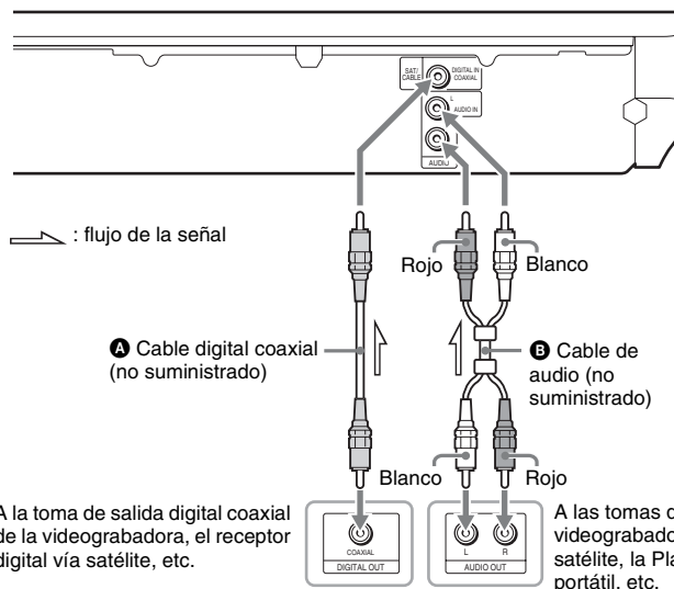
Panel posterior de la unidad
