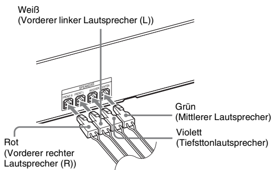
Rückseite des Geräts
