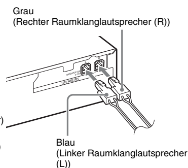
Rückseite des Raumklangverstärkers
