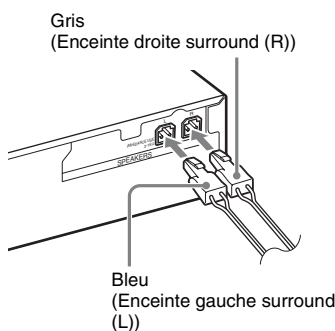
Panneau arrière de l'amplificateur surround
