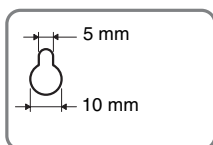
Foro sul retro del diffusore
