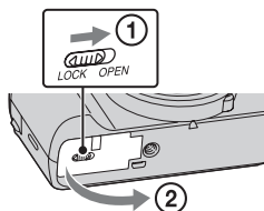
Palanca de expulsión de la batería
