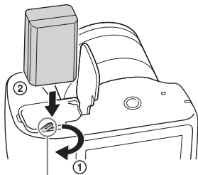
Vergrendelingshendel
