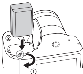
Dźwignia blokady
