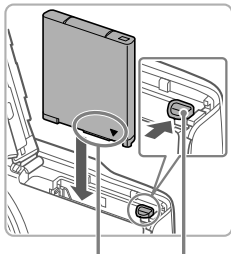
Anschlüsse Akkuverriegelung
