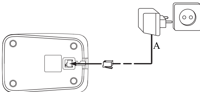
- 2C. Kézibeszélő - A. Adapter tápkábellel
