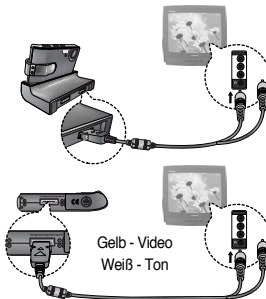
[AV-Kabel mit Basisstation verwenden]
