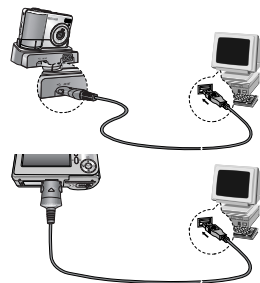
[Einsatz des USB-Kabels mit der Basisstation(Sonderzubehör)]
