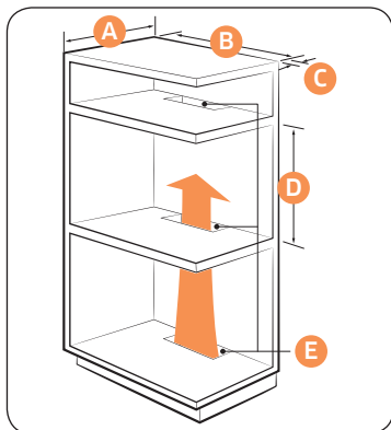
Einbauschrank (mm)
