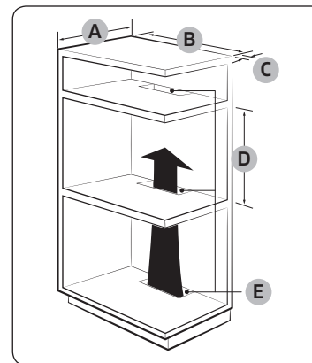
Einbauschrank (mm)
