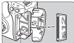
CF-Karte Auswurf-taste
