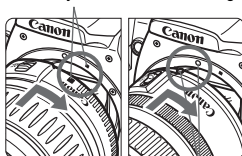
EF-Objektivansetz-Markierung
