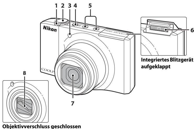
Objektivverschluss geschlossen
