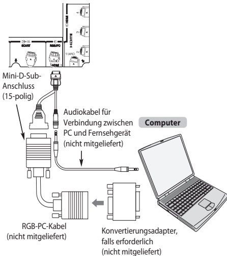
Rückseite des Fernsehgeräts
