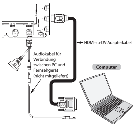
Rückseite des Fernsehgeräts
