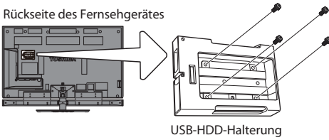
USB-HDD-Halterung
