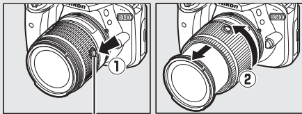
Tubusverriegelung
