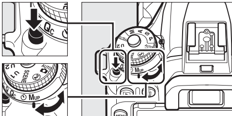
Aufnahmebetriebsartenwähler
