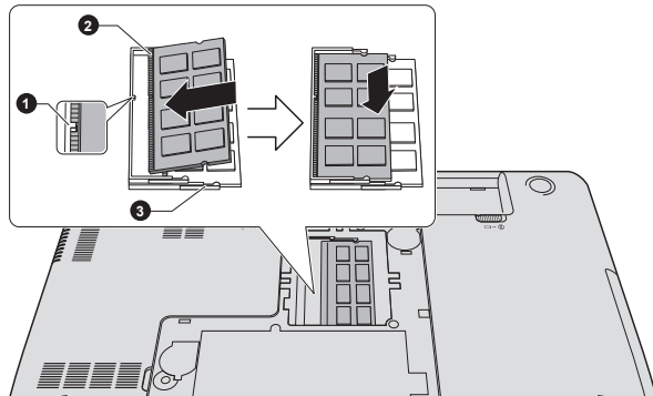
Abbildung 4-12 Speichermodul einsetzen
