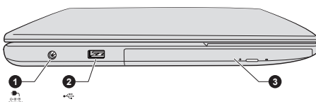
Abbildung 3-2 Linke Seite des Computers
