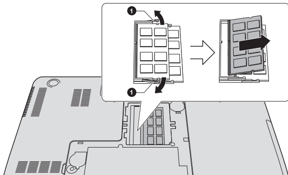
Abbildung 4-14 Speichermodul entfernen
