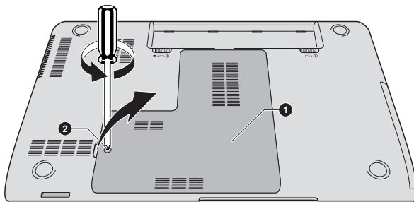
Abbildung 4-11 Speichermodul-Abdeckung entfernen
