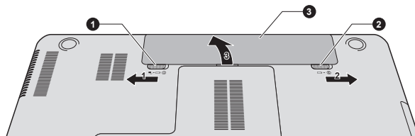
Abbildung 4-9 Akku entsichern -1
