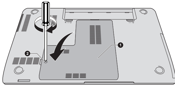
Abbildung 4-13 Speichermodulabdeckung einsetzen
