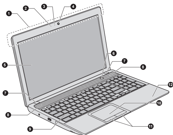
Abbildung 3-6 Vorderseite des Computers mit geöffnetem Bildschirm
