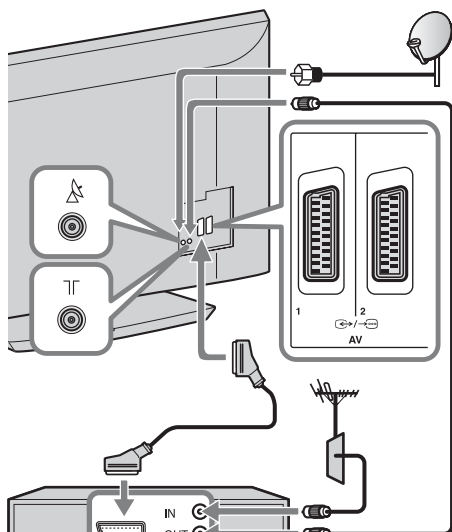
Décodeur/graveur (de DVD, par exemple)
