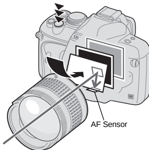
AF Sensor
