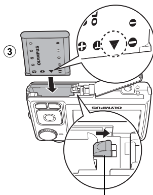
Akkuverriegelung
