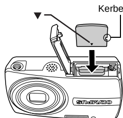
Akku-/Kartenfachdeckel
