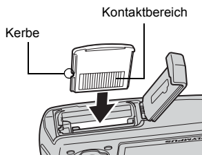
Akku-/Kartenfachdeckel
