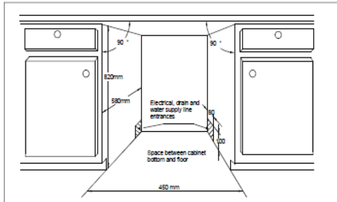
[Abb. 1] Abmessungen des Unterbaus: Weniger als 5 mm Platz zwischen Oberkante des Geschirrspülers und des Unterbaus und der zum Unterbau ausgerichteten Tür.
